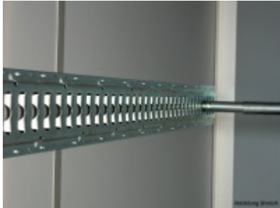
Ankerschienen mit Sperrstange
